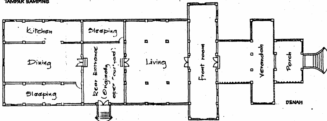
Gb.8. Tipe Rumah Kepala Kampung Malaka Abad ke-15. SUMBER: S. VLATKAS, 1990: 16.
