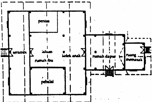
Gb.11. Rumah Bumbung Panjang Pahang SUMBER: NASIR & WAN TEH, 1994: 40
